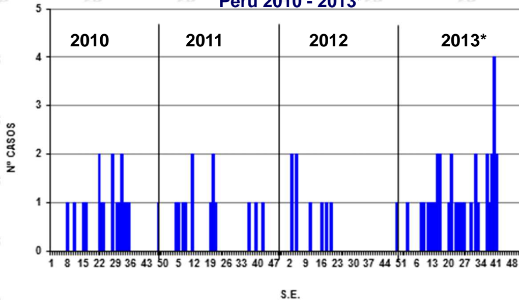
Casos de fiebre amarilla por semana. Perú 2010 - 2013*
