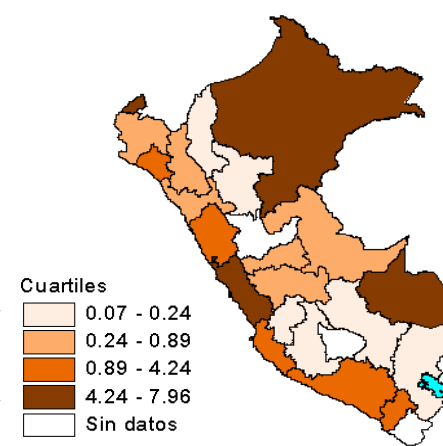
Incidencia acumulada 2009
