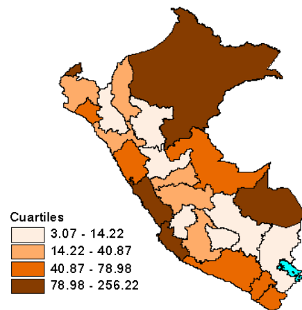
Incidencia acumulada 1983 - 2008
