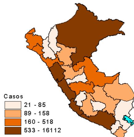
Casos acumulados 1983 - 2008
